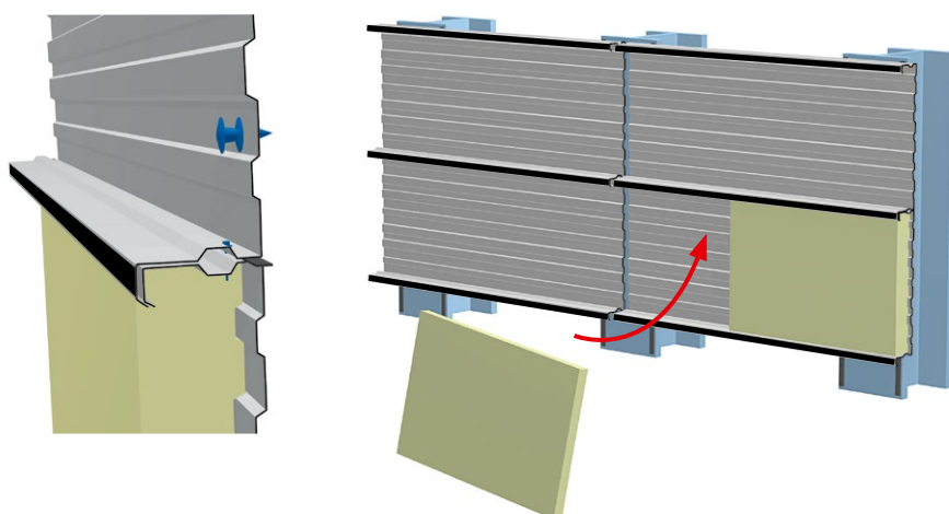
Docieplenie standardową wełną mineralną.
