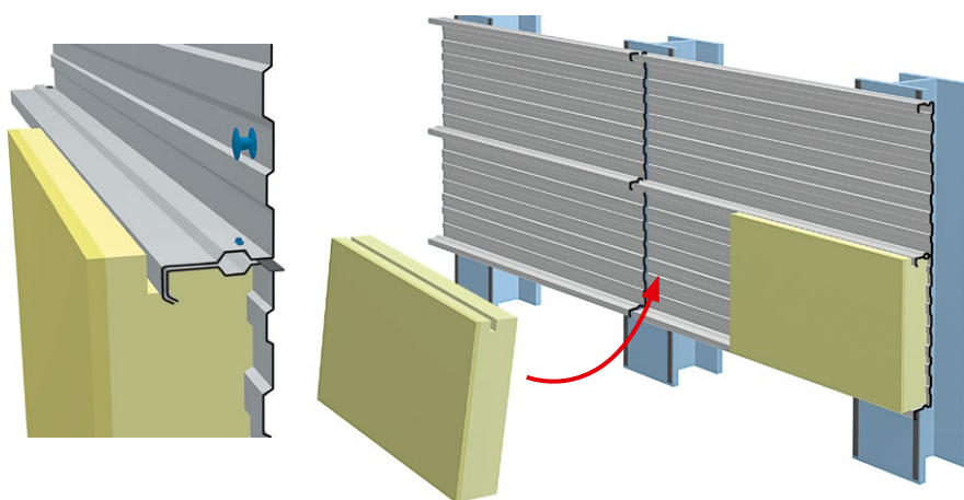
Docieplenie dwugęstościową wełną skalną ze żłobieniem.
