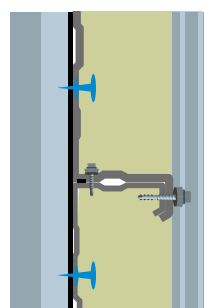
Łącznik samowiercący 5,5 x 19 mm
