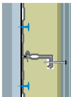
Dystansowy łącznik samowiercący 5,5 x 63 mm
